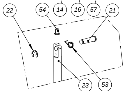
DETALLE B
