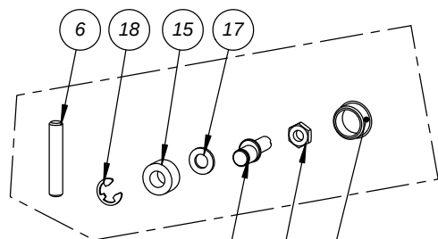
DETALLE A
